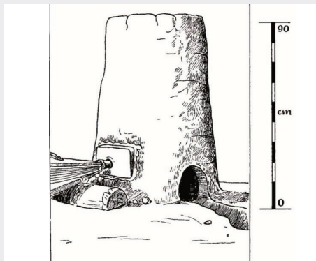
Kresebná rekonstrukce železářské pece
